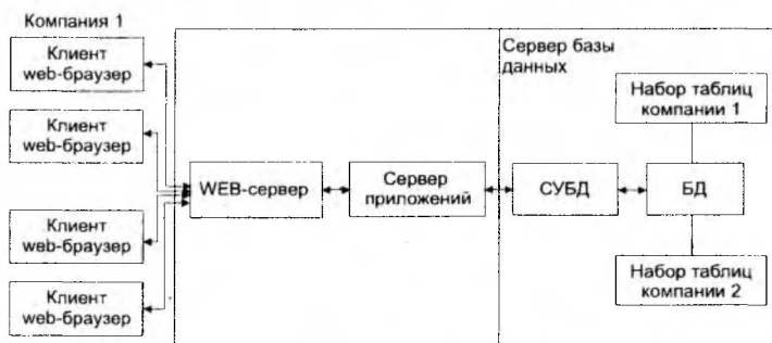
Структура ASP-провайдера
